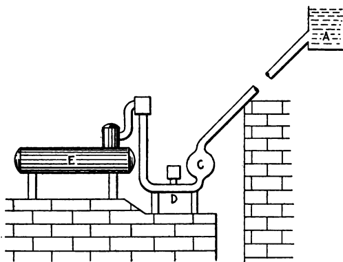
FIG. 3.—Sommeiller's compressor.
